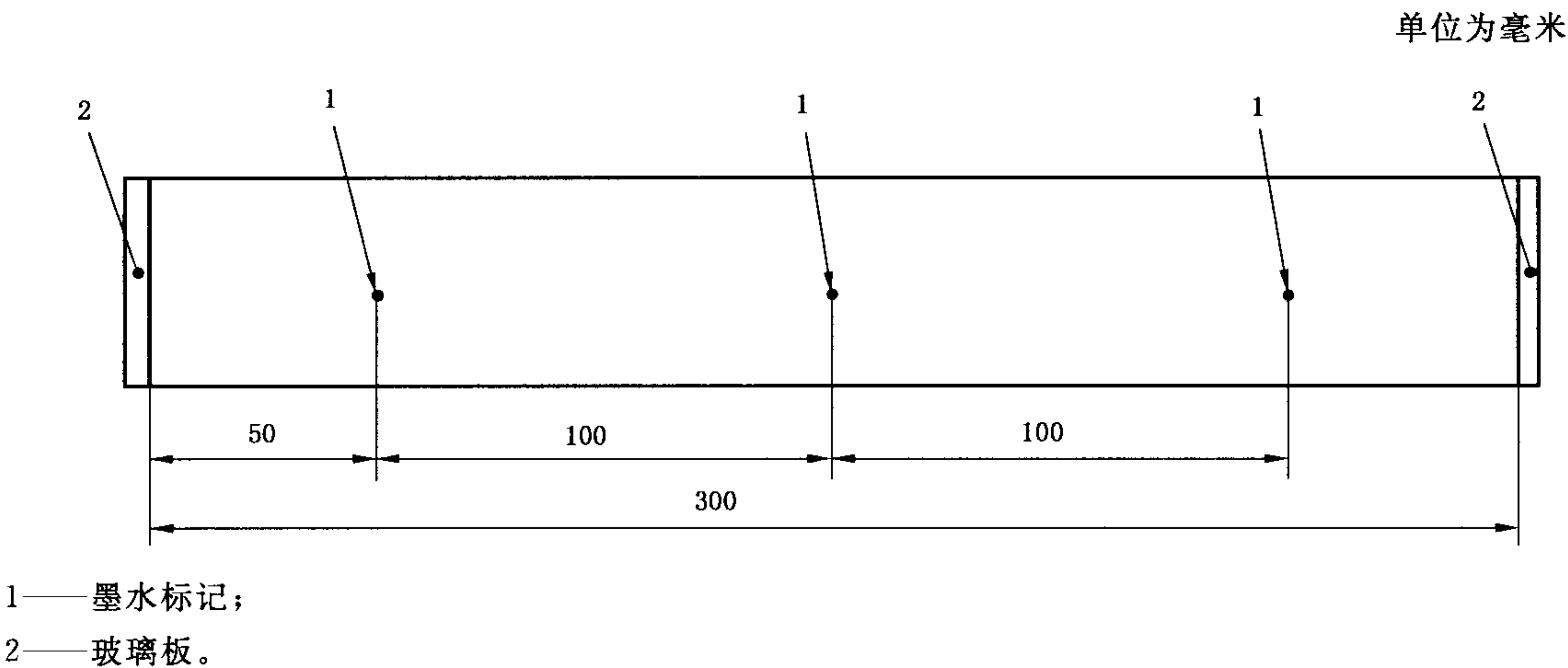
图 13 厚度测量点示意图
