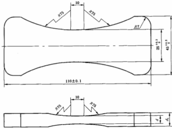
图 3 III 型试样型式
