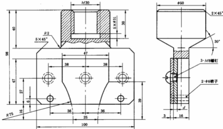
图 5 III 型试样使用的夹具
