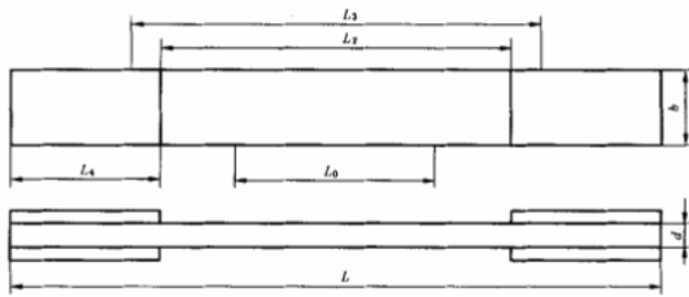
图2 II型试样型式
