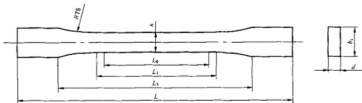
图 1 I 型试样型式
