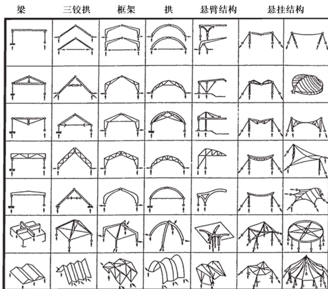
图3.1 木结构体系：梁、三铰拱、框架、拱、悬臂结构、悬挂结构 (Winter, 2004)
