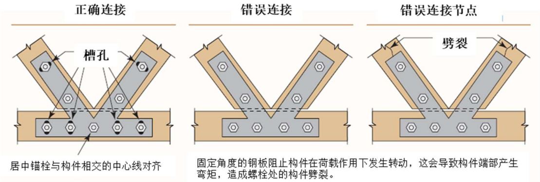
图 3.9 桁架连接节点（图片由 APA 提供）
