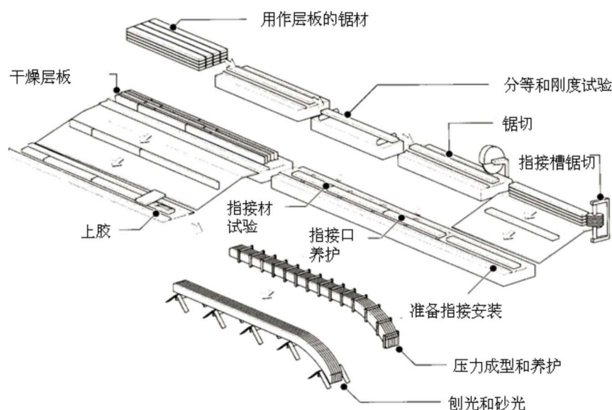
图 1.1 胶合木加工生产过程示意图
