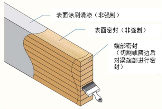
图 5.10 梁端密封处理示意图
