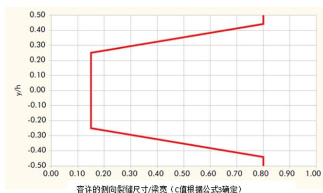
图 5.5 容许侧向裂缝深度
