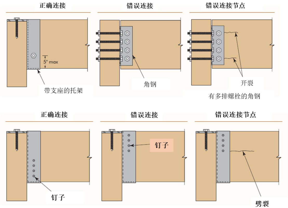
图 3.5 梁与梁的连接（图片由 APA 提供）
