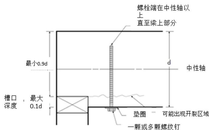
图 5.6 推荐的受拉侧槽口增强方式
