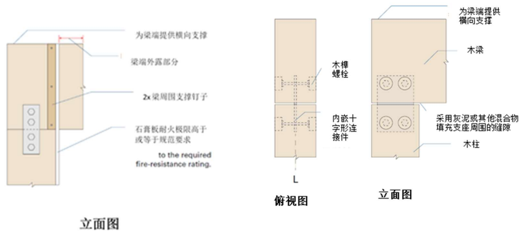
图 4.4 隔离式梁柱连接节点构造
