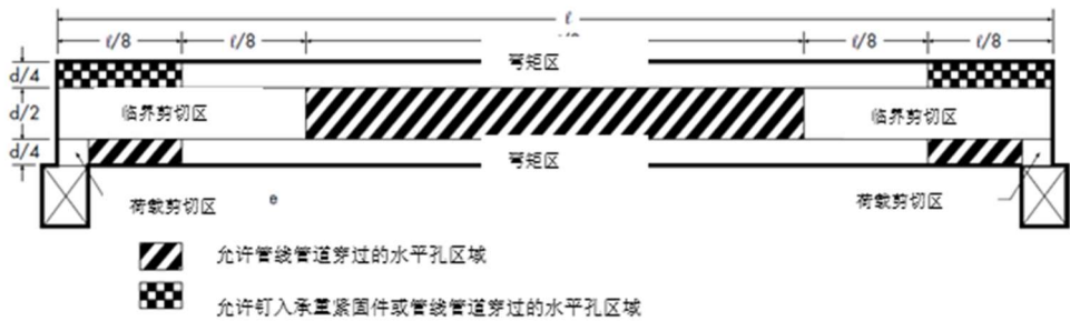
图 5.8 均布荷载作用下简支梁水平孔位置
