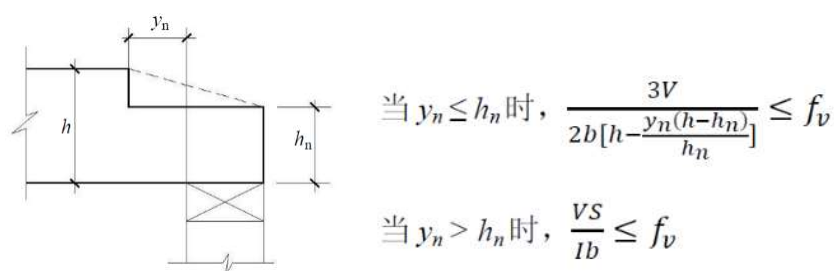
图 5.7 受弯构件端部受压边槽口剪切强度设计公式
