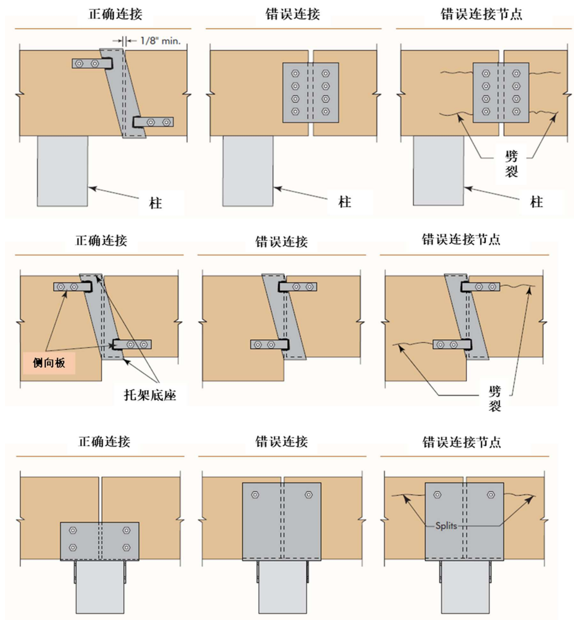
图 3.7 悬臂梁连接-无拉伸约束（图片由 APA 提供）
