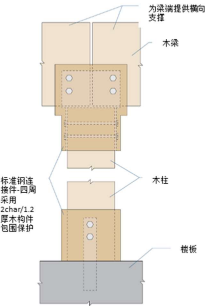
图 4.7 包覆式柱与柱连接节点构造
