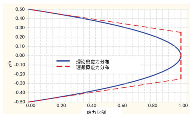
图 5.4 理论与理想剪应力分布图
