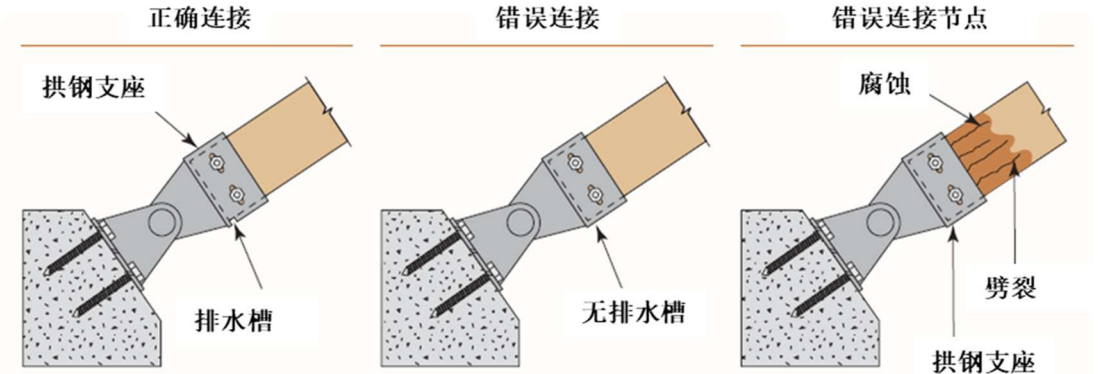
图 3.10 胶合木拱与基础的连接（图片由 APA 提供）
