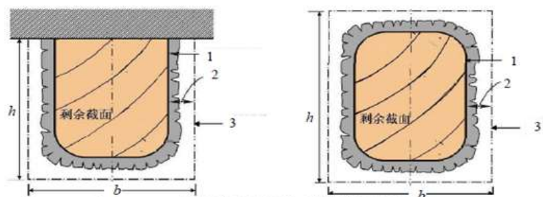
图 5.1 三面曝火和四面曝火构件截面简图
