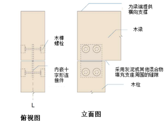
图 4.5 外露式梁柱连接节点构造（有外观要求）
