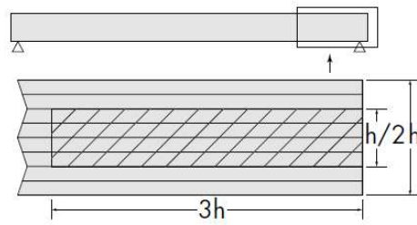
图 5.2 胶合梁端部临界剪切区
