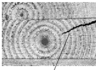
图 5.1 胶合木干裂
