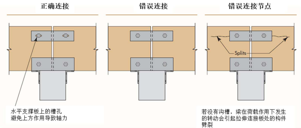
图 3.8 梁柱-U 型支架-木材或管柱（图片由 APA 提供）
