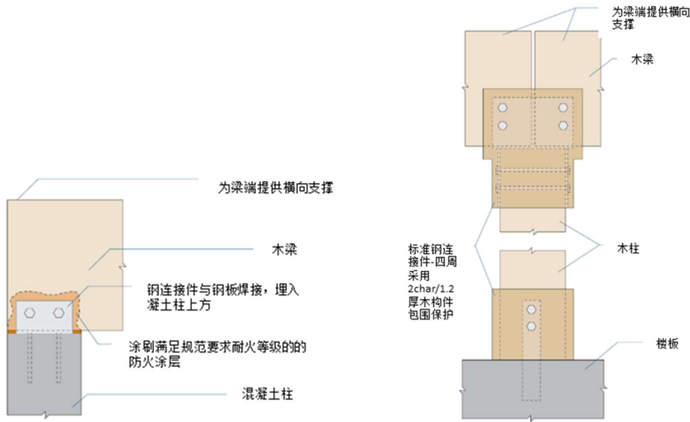
图 4.6 外露式梁柱连接件节点构造（无外观要求）
