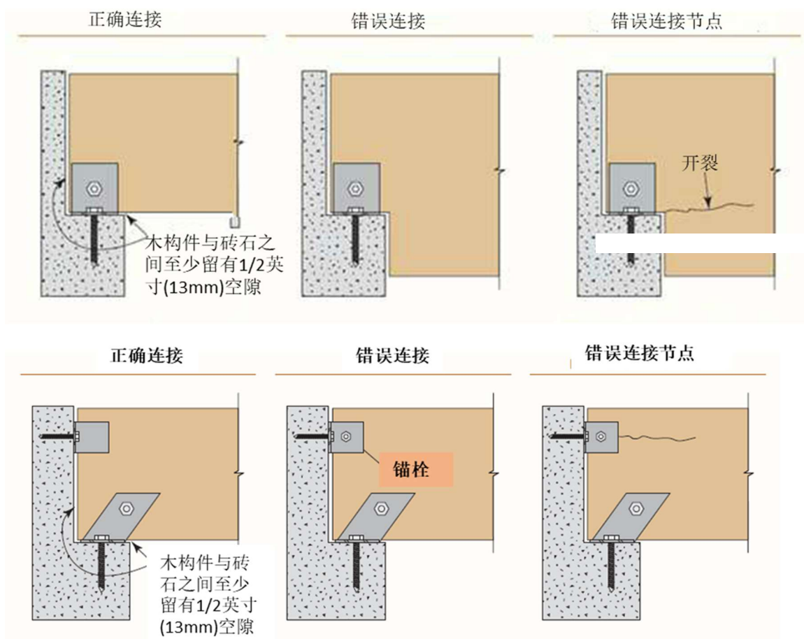
图 3.4 梁与支座的连接（图片由 APA 提供）
