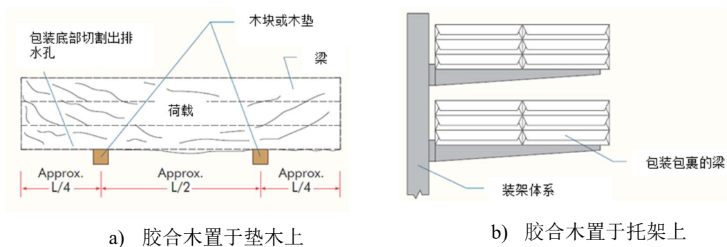
图 5.9 胶合木场地存放示意图
