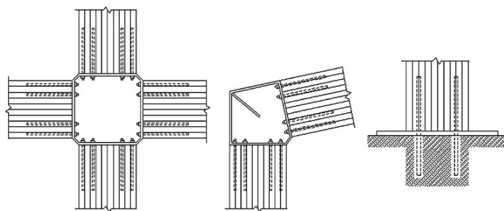
图 3.3 植筋连接应用示意图
