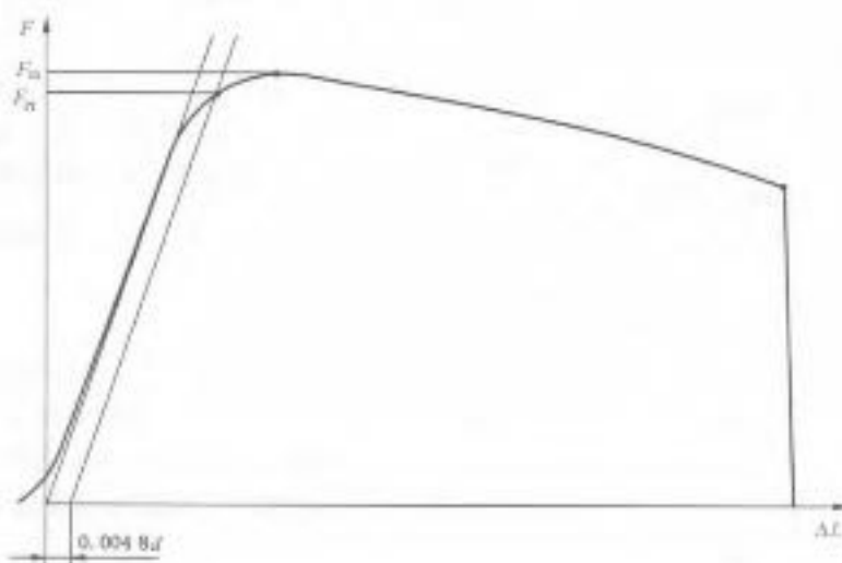
图 4 测定 0.004 8d 非比例延伸应力 R_{p0.0048d} 的载荷-位移曲线
