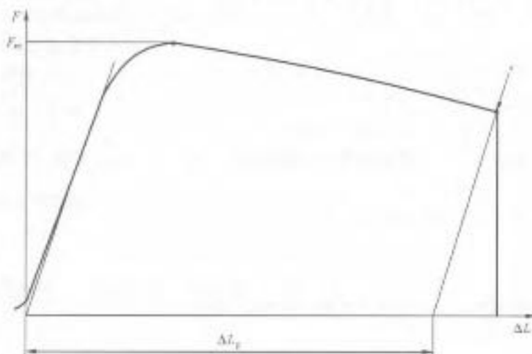
图 3 测定断后伸长率 A_t 的载荷-位移曲线
