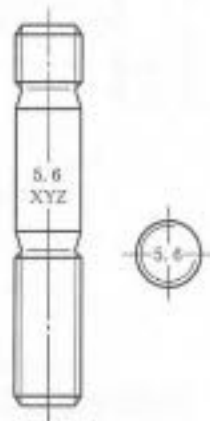
图 14 螺柱标志示例
