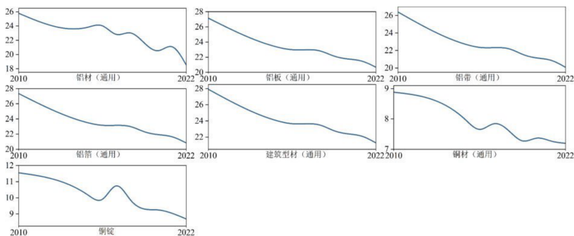
图 S2.10 2010-2022 年有色金属产品排放因子
