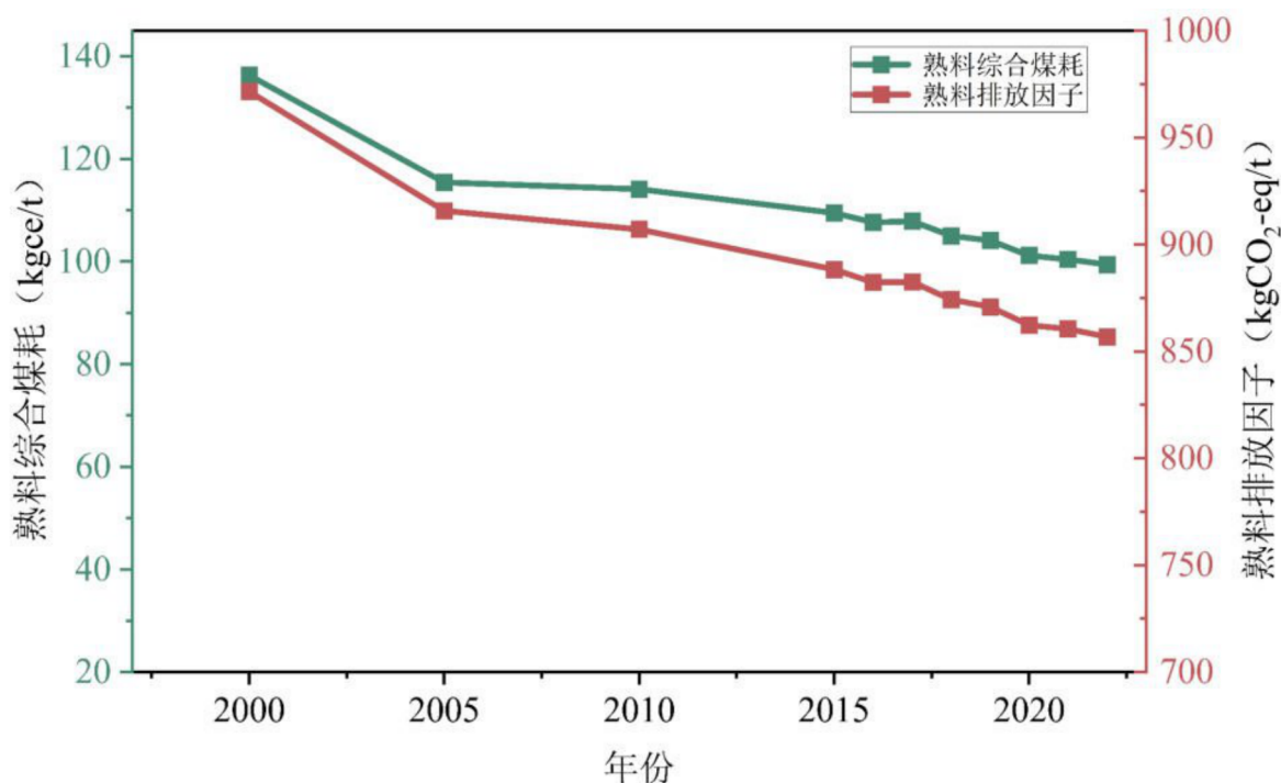
图 S2.2 2000-2022 年熟料综合煤耗及排放因子
