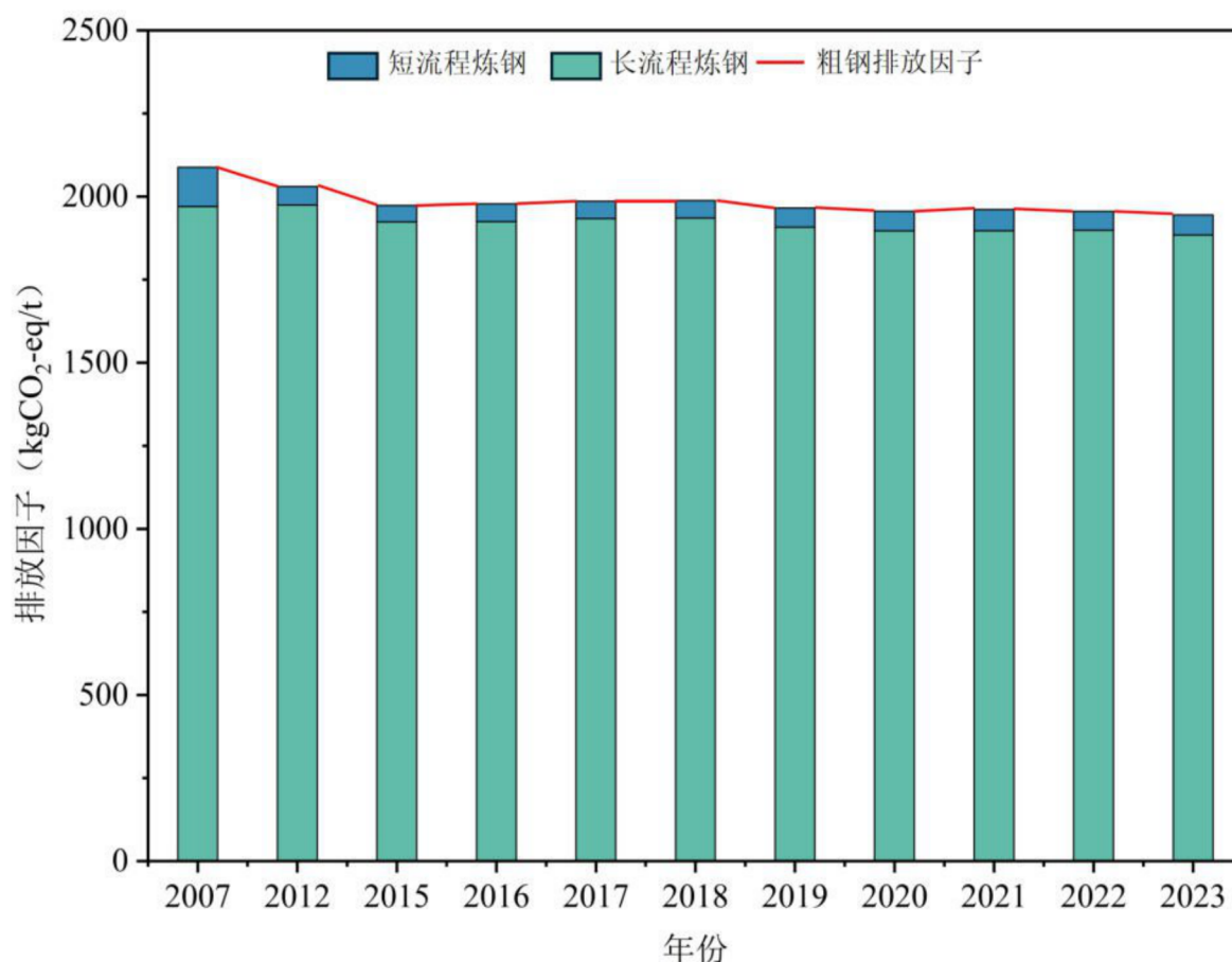
图 S2.4 2007-2023 年粗钢排放因子及排放结构
