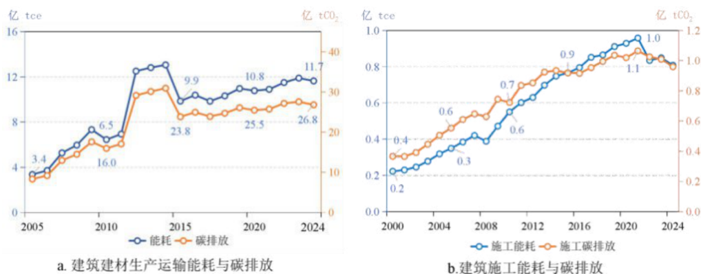
图 1.3 建筑建造能耗与碳排放变化趋势
