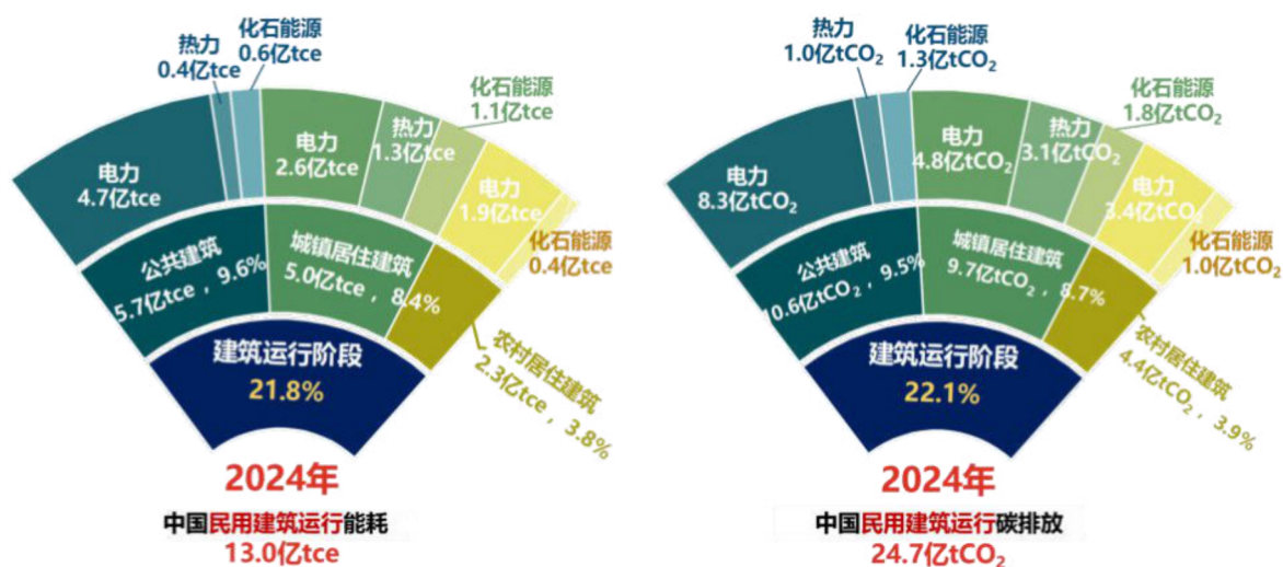
图 1.4 2024 年全国民用建筑运行能耗与碳排放
