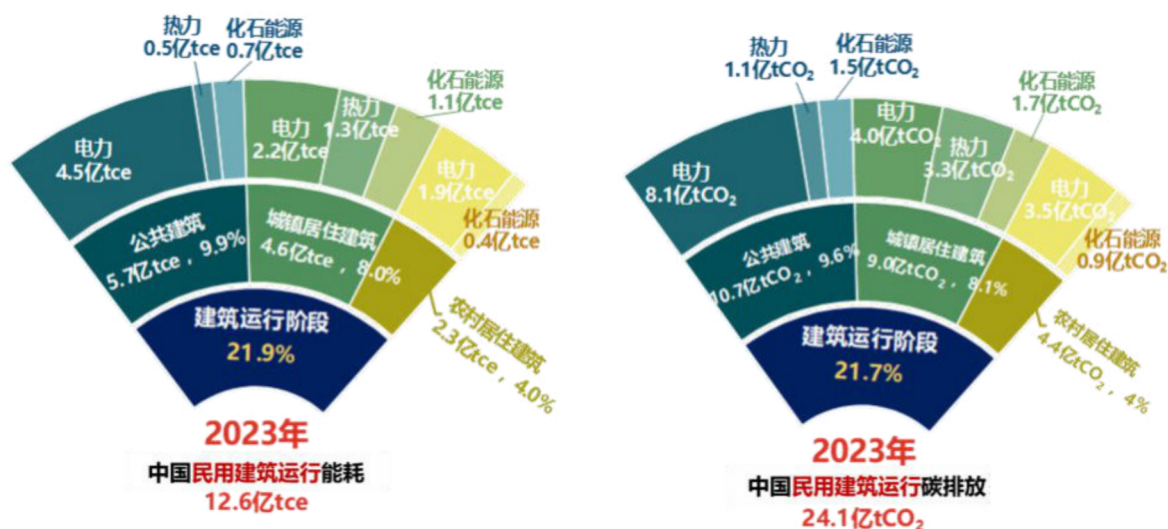
图 1.5 2023 年全国民用建筑运行能耗与碳排放
