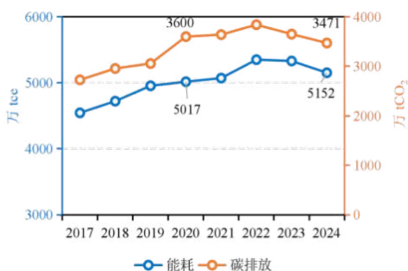
b. 土木工程施工能耗与碳排放
